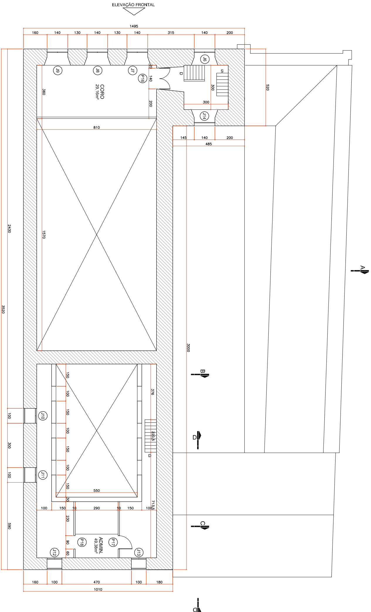
PLANTA PAVIMENTO SUPERIOR Escala 1:150
